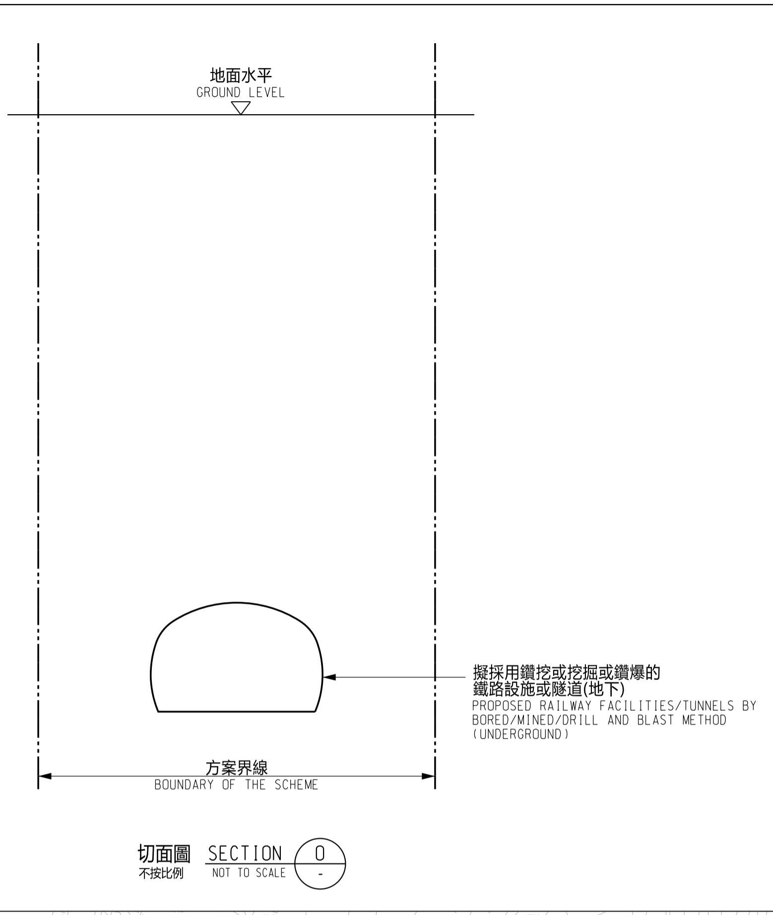
切面圖 SECTION 0 不按比例 NOT TO SCALE
